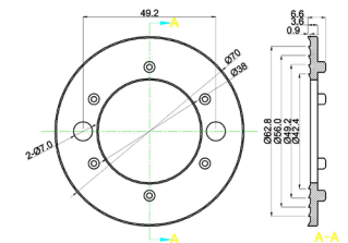
Bottom Gasket
